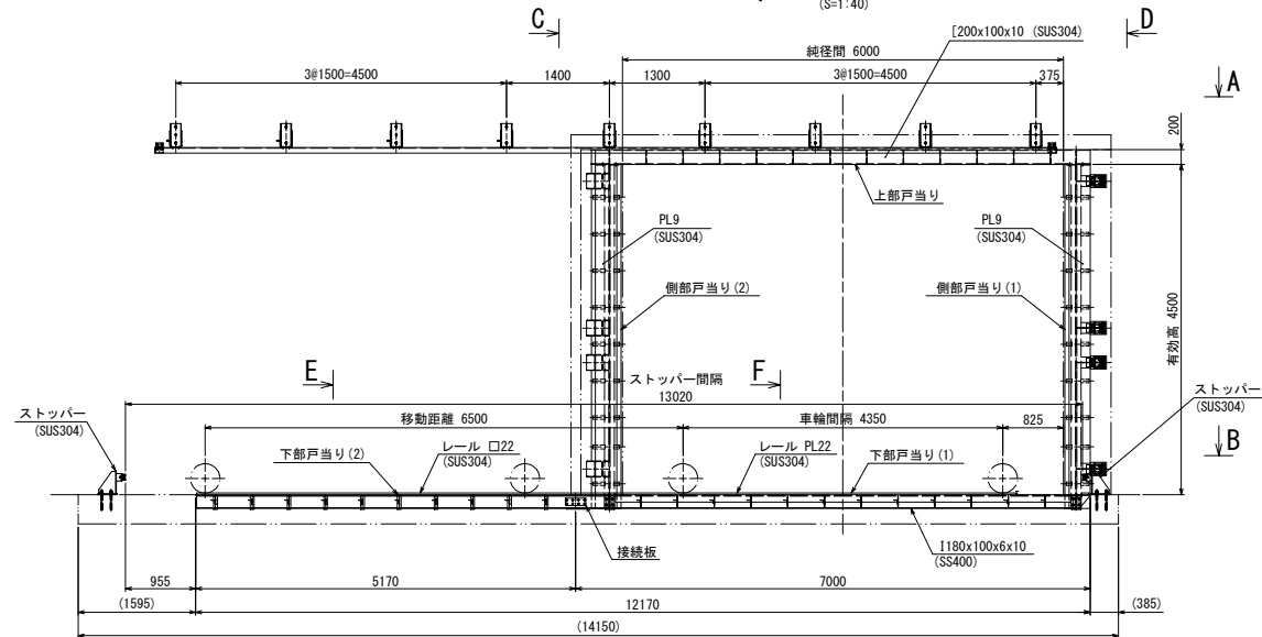
正面図 (S=1:40)
