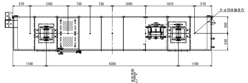
E 矢視
