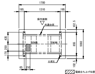
基礎及び電線立上がり位置図
