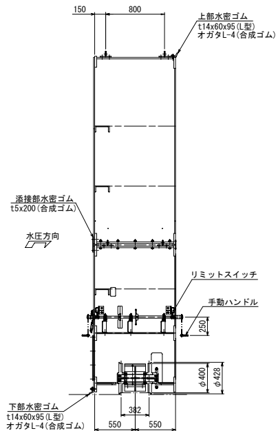
C 矢視
