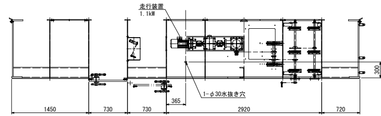
I 矢視
