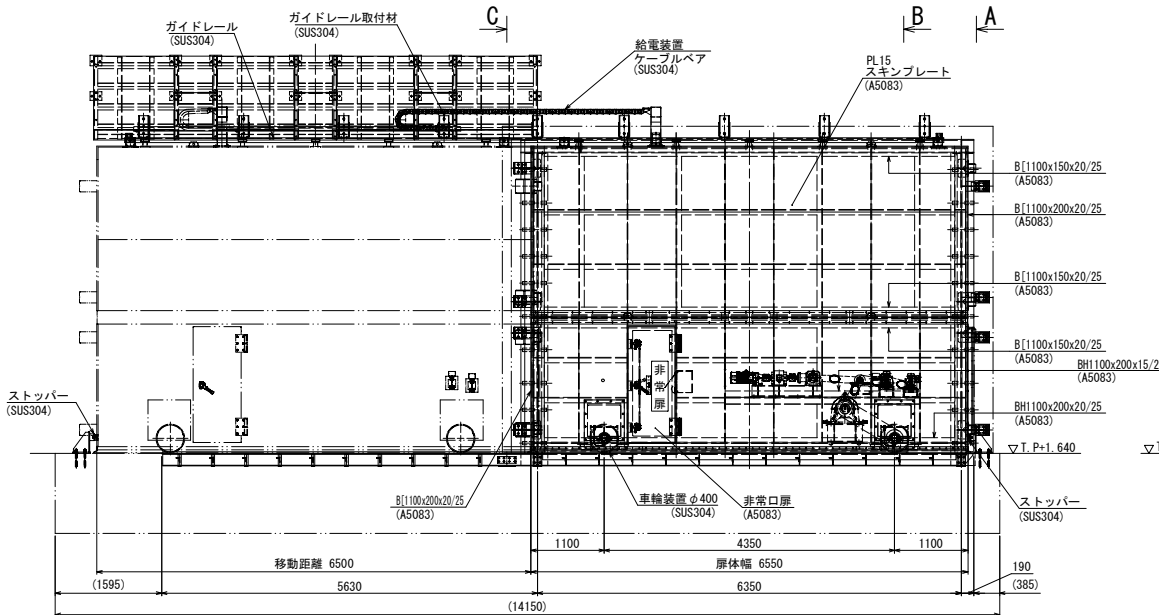
正面図 (S=1:40)
