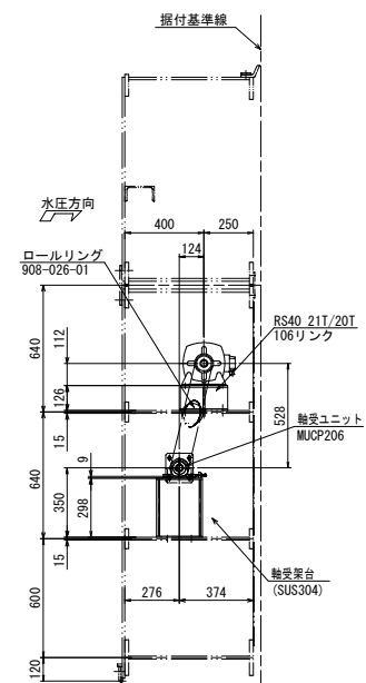
D 矢視
