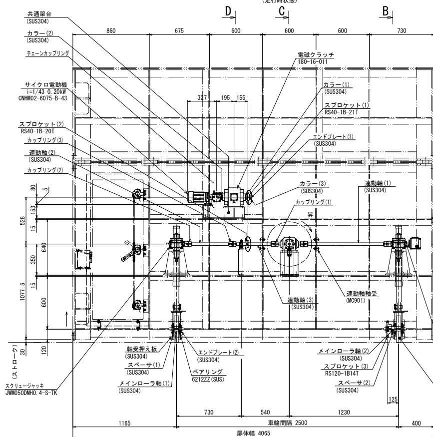
正面图
