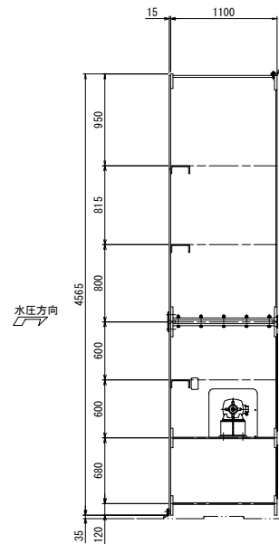
E 矢視
