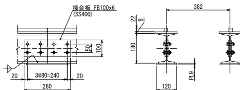
現地接合部詳細 (S=1:8)
