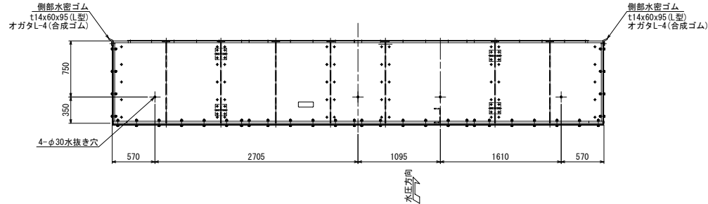
C 矢視
