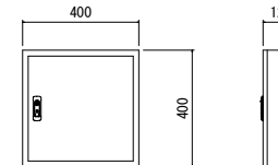
接地端子盤 S=1:10
