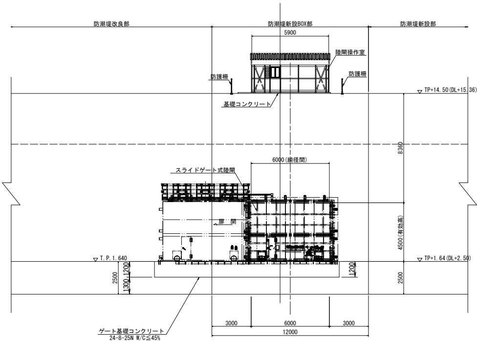
平面図
