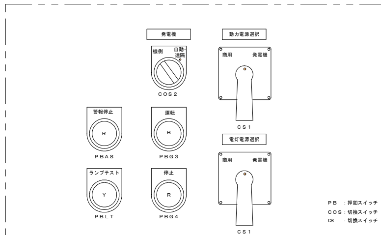
中扉詳細
