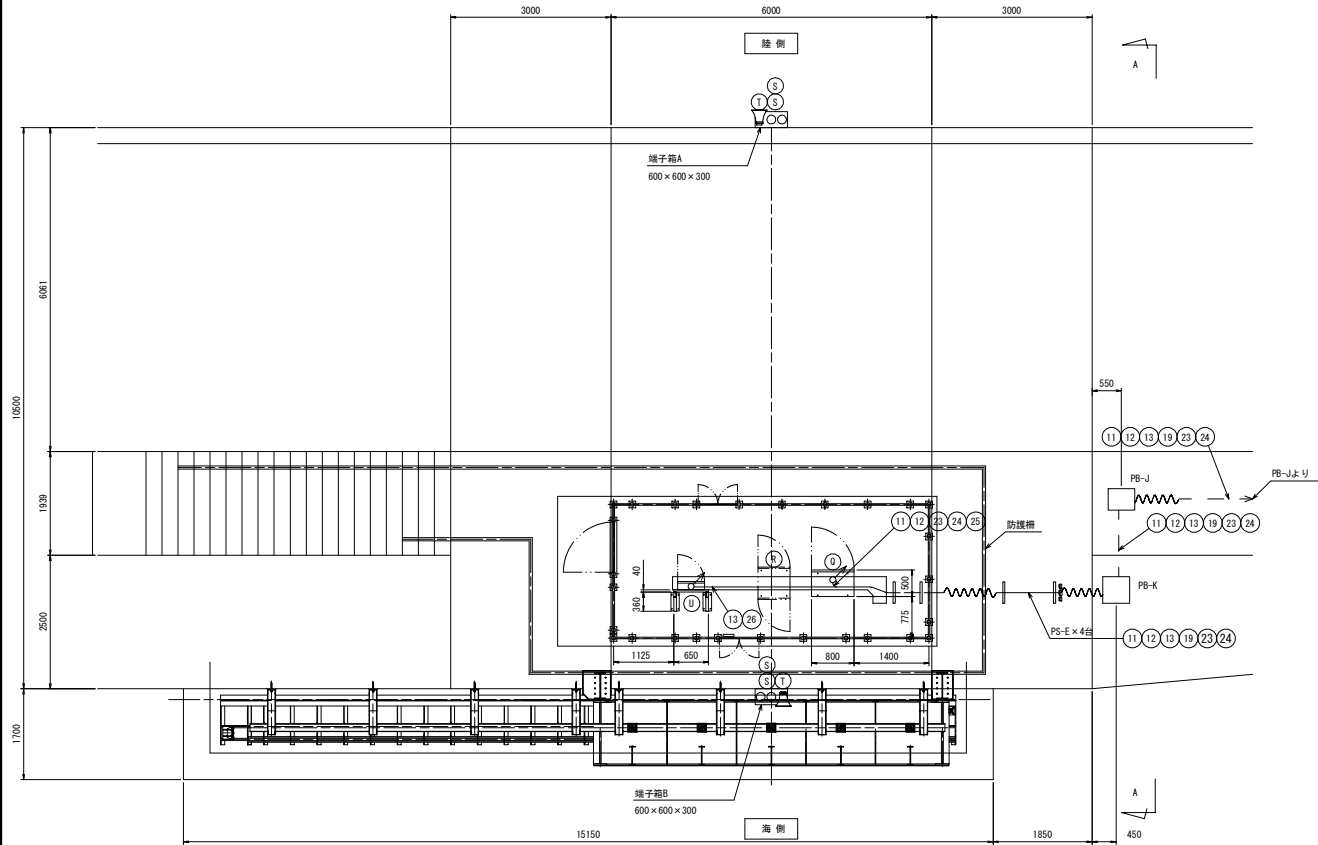
盤取付け架台図(参考図)
