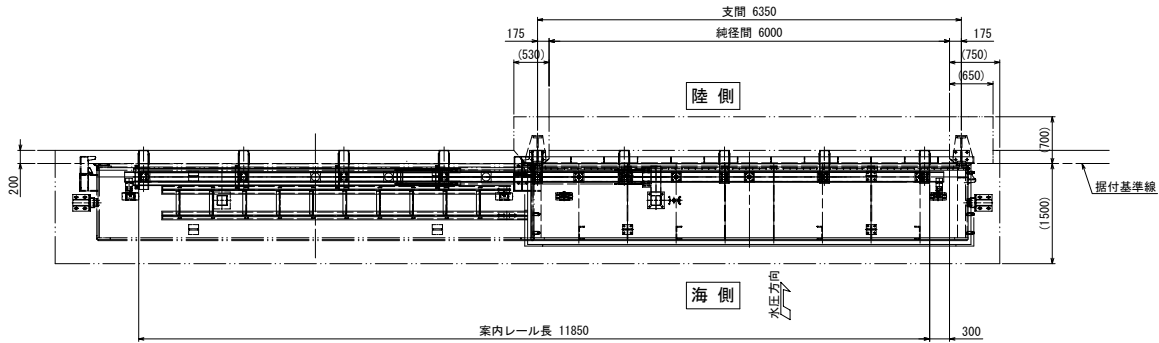
平面図 (S=1:40)
