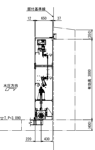
B 矢視
