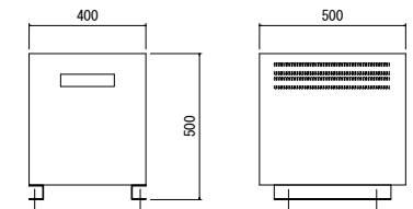
耐雷トランス S=1:10
