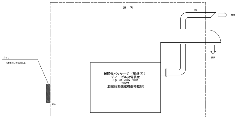
配管フロ一図
