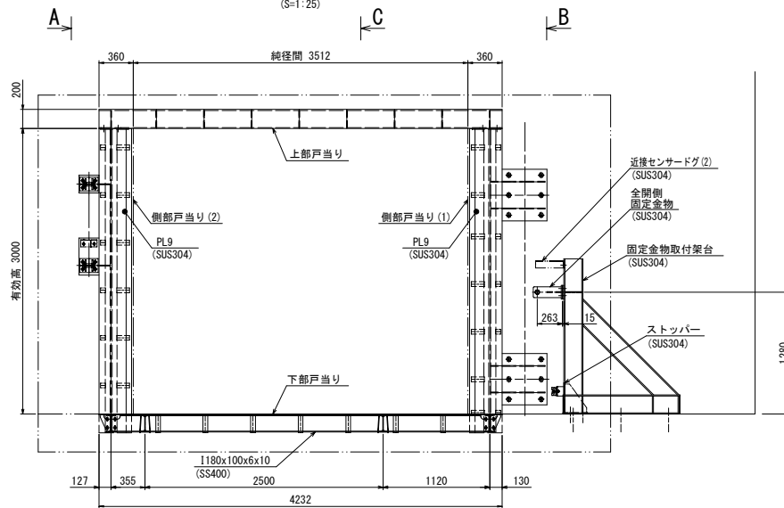
正面図 (S=1:25)
