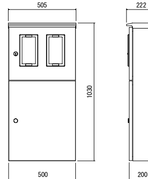
引込開閉器盤 外形図 S=1:10
