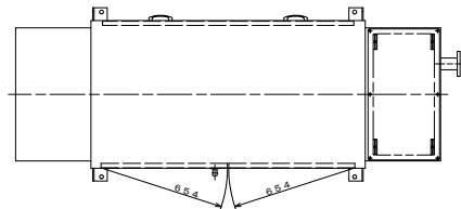
予備発電機 外形図 S=1:15
