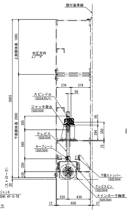
B 矢視
