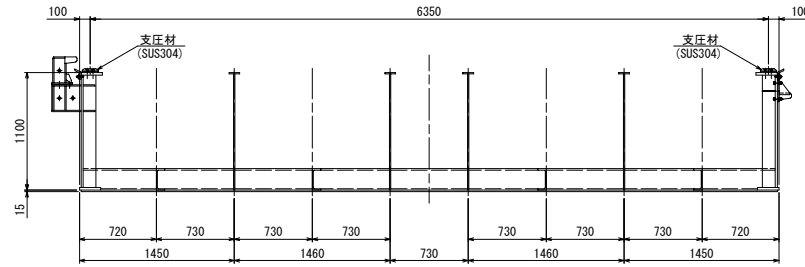
G 矢視
