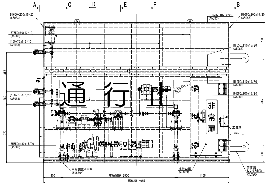
正面図 (S=1:15)
