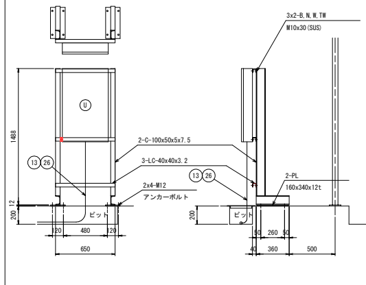
盤取付け架台図(参考図)
