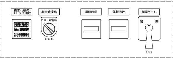
機側操作盤中扉詳細
