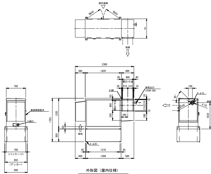
外形図（屋内仕様）
